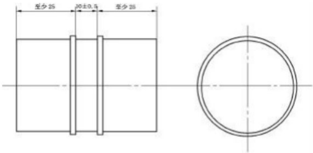
图 A.2 带导电涂层的管和棒状试样
