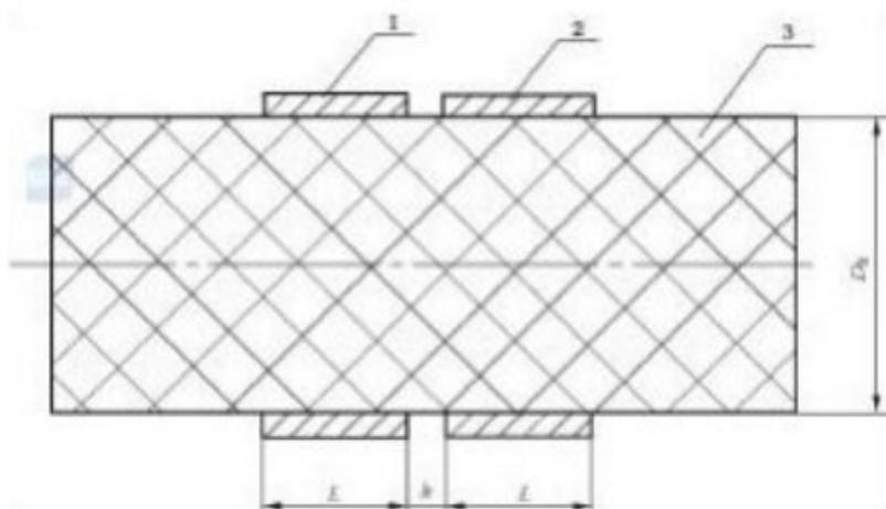
图 2 管状试样电极配置
